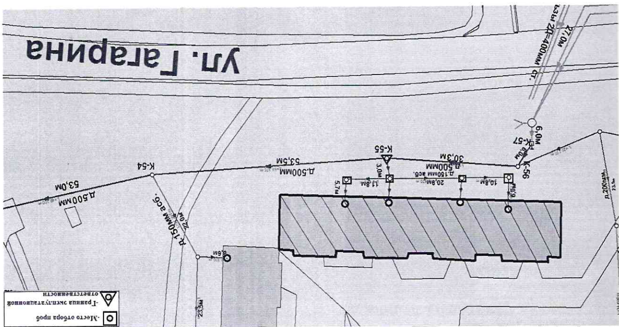
Схема водопотребления: По адресу: ул. Рубжаная, д. 29 корп. 2
