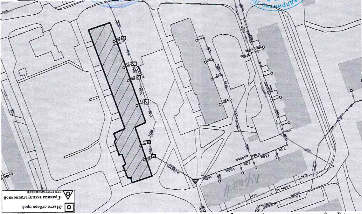
По адресу: Б. Каменная, д. 9 корп.4 Схема водоотведения:
